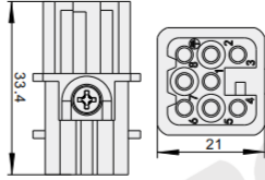
X901-8F 母插体
