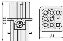
X901-7F 母插体
