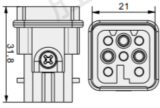
X901-8M 公插体
