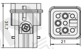
X901-7M 公插体
