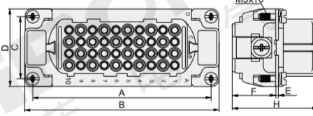
母插体
