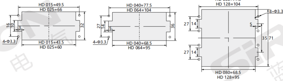
面板安装开孔图
