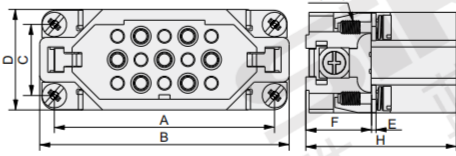
公插体
