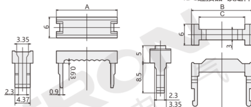
IDC连接器-锁定位
