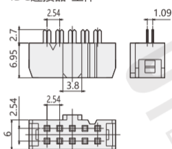
IDC连接器-主体
