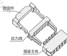
IDC连接器-锁定位
