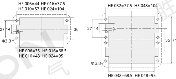
面板安装开孔图
