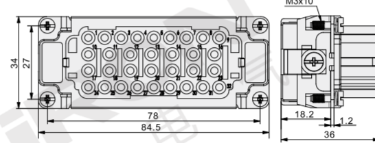
X906-46F 母插体
