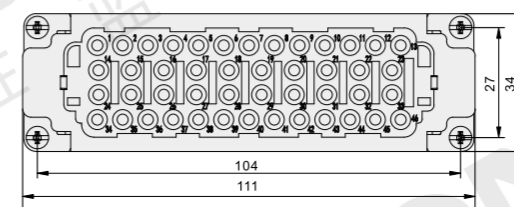
X906-46F 母插体
