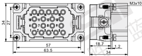
X906-32M 公插体
