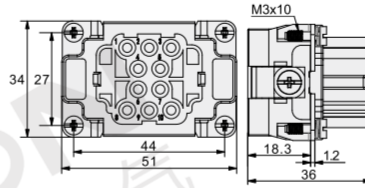
X906-18F 母插体
