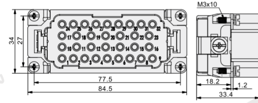
X906-46M 公插体
