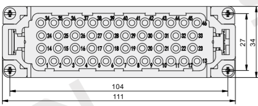
X906-46M 公插体
