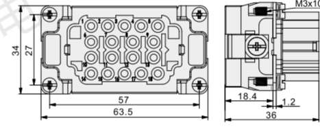
X906-32F 母插体
