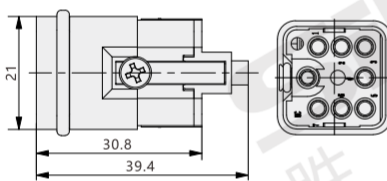
X907-12M 公插体
