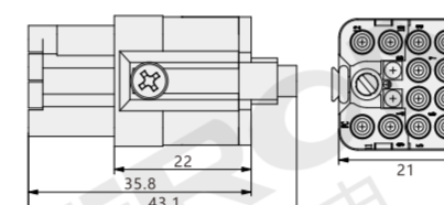
X907-12F 母插体
