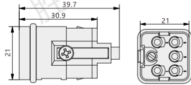
X907-7M 公插体
