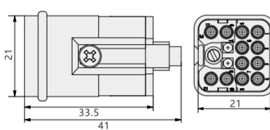
X907-12M 公插体
