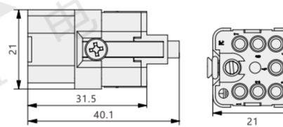
X907-12F 母插体
