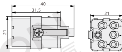
X907-7F 母插体
