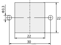
面板安装开孔图
