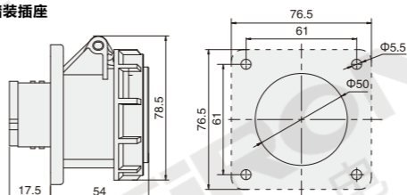
暗装插座
