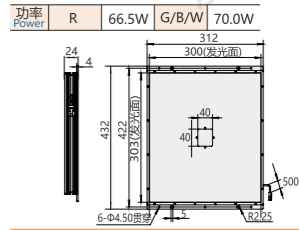
K716Z-400300(中孔型) mm
