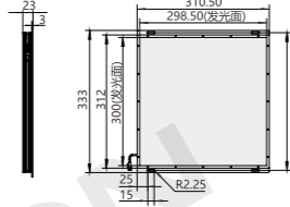
K716Z-150100(中孔型) mm
