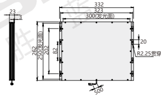
K716Z-12080(中孔型) mm
