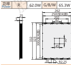
K716Z-300250(中孔型) mm
