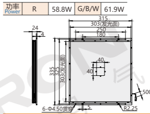
K716Z-300300(中孔型) mm
