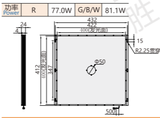
K716Z-400400(中孔型) mm
