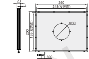
K716Z-250190(中孔型) mm
