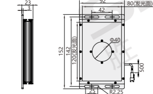
K716Z-200160(中孔型) mm
