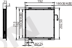
K716-200200 mm
