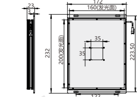
K716Z-200160(中孔型) mm
