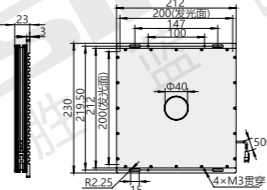
K716Z-200200(中孔型) mm
