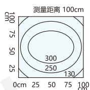
亮度分布图 基于10W实例灯具 测量单位:lx
